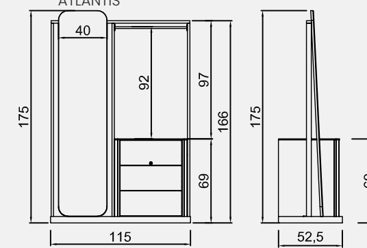
DRESSER ATLANTIS
