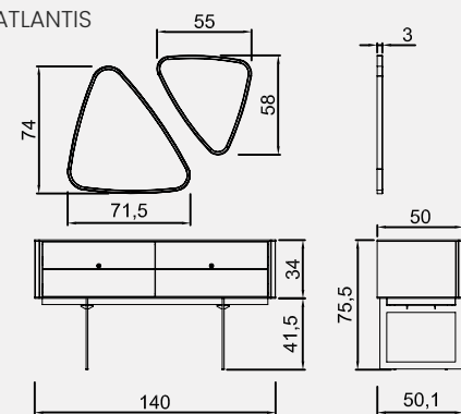
DRESSER ATLANTIS
